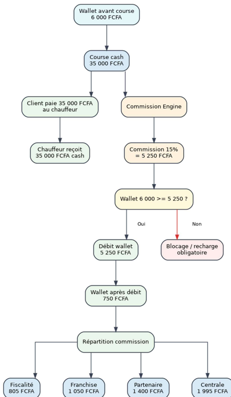
Figure 2 - Exemple de contrôle wallet avant débit de commission
