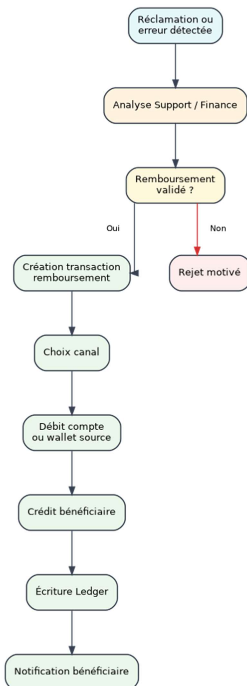
Workflow - 62. Use case 14 - Remboursement client, chauffeur ou partenaire
