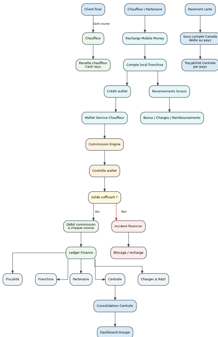
Figure 3 - Architecture financière globale du module Finance
