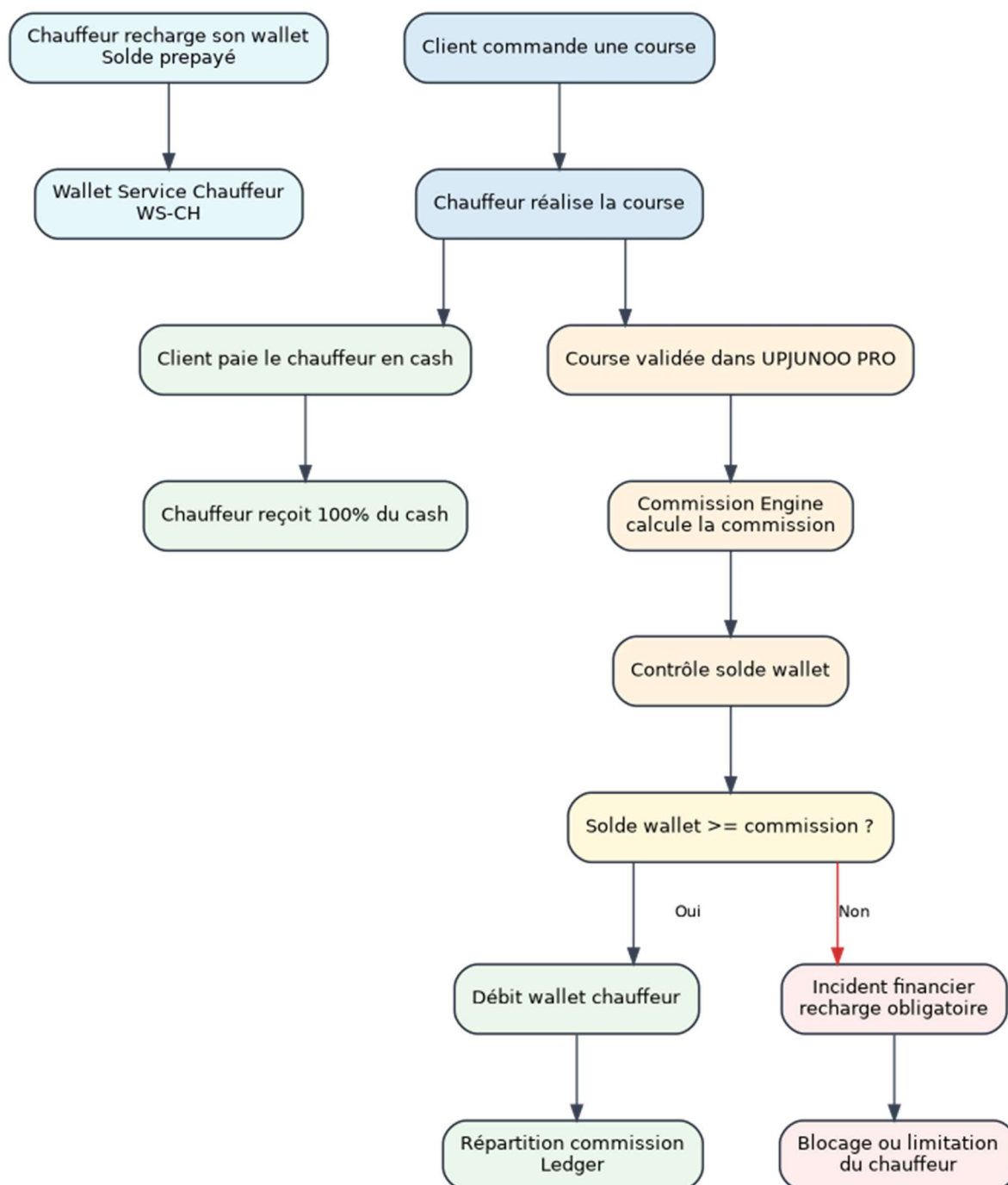
Figure 1 - Schéma du modèle prépayé UPJUNOO PRO
