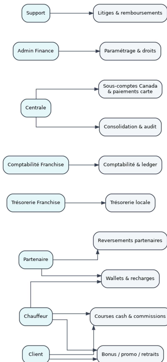
Figure 6 - Diagramme global des cas d'utilisation du module Finance
